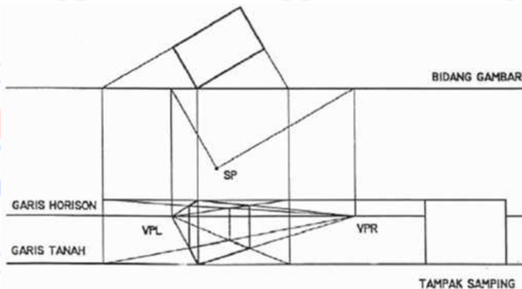
Gambar 4.71 Perspektif 2 Titik Hilang Tipe A
