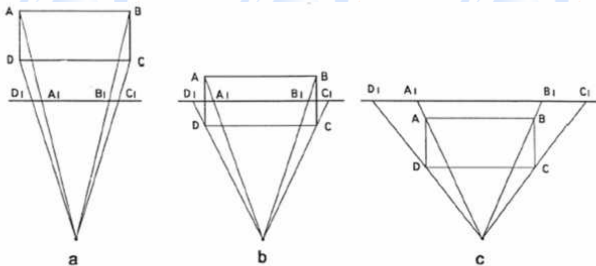
Gambar 4.66 Peletakan Bidang Gambar
