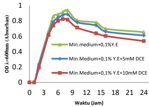
Gambar 1 Kurva Pertumbuhan Pseudomonas aeruginosa pada 0-24 jam
