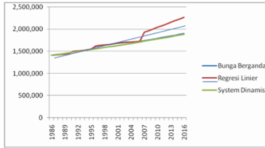
Gambar 4 Grafik Perkembangan Jumlah Penduduk Tahun 1986 s/d 2016 dengan Model Regresi Linier, Bunga Berganda dan System Dinamis
