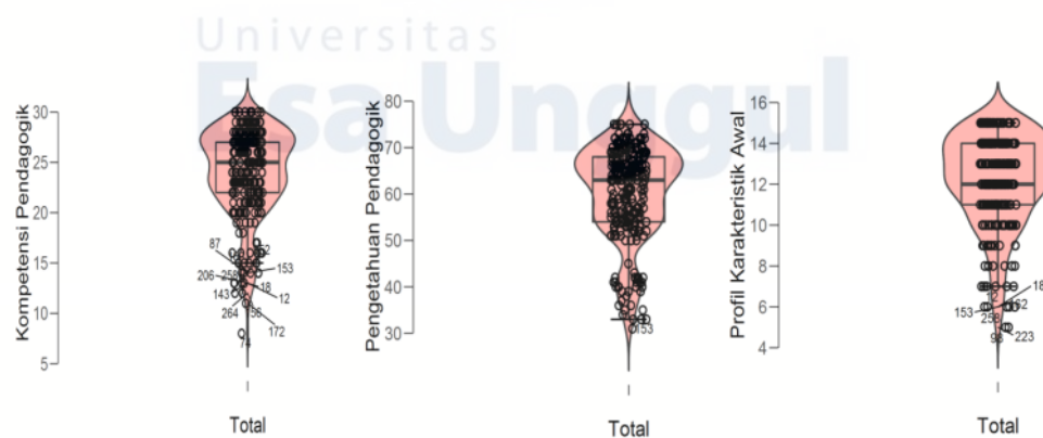
Gambar 1. Boxplot variabel kompetensi pedagogik, pengetahuan pedagogik, dan profil karakteristik awal
