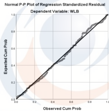
Gambar 1 Uji Normalitas
