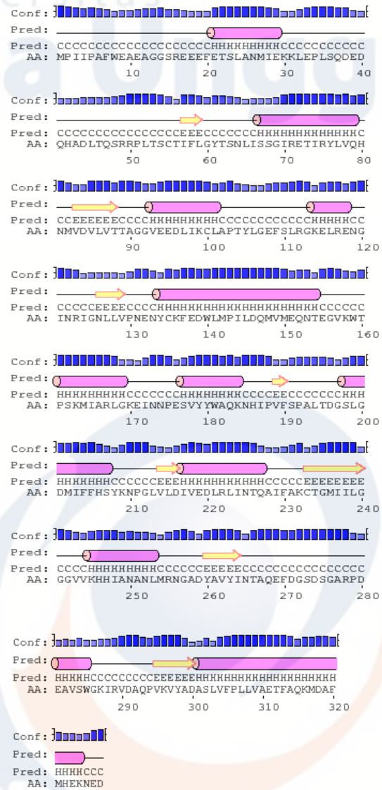
Gambar 3. Struktur Sekunder Pada Protein DHPS Normal Dan Mutan
