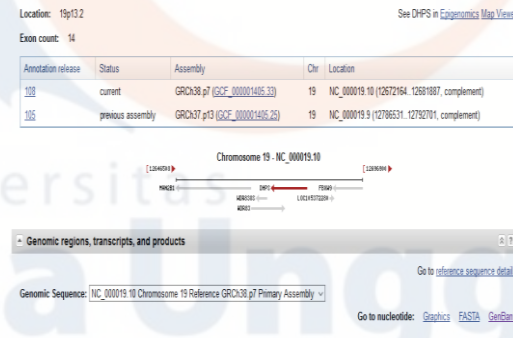
Gambar 1 Lokasi Gen DHPS
