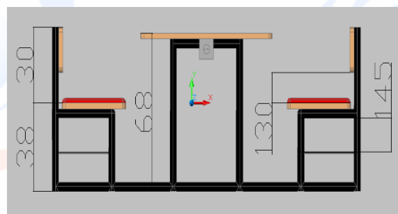
Gambar 6. Desain Meja dan Bangku Tampak Samping
