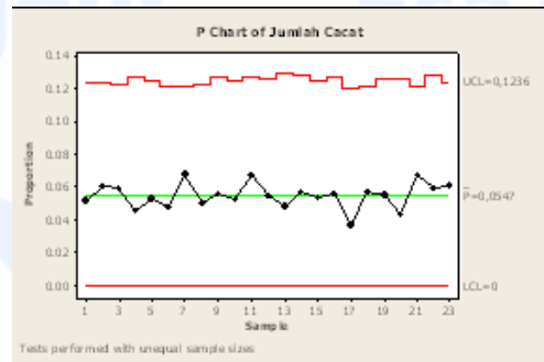
Gambar 2 P-Chart Produk Cacat Pada Proses Viskositas
