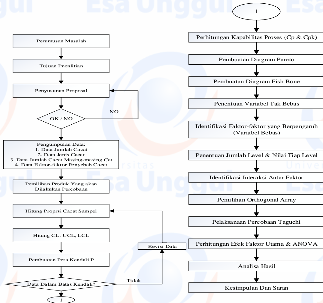
Gambar 1 Alur Tahapan penelitian
