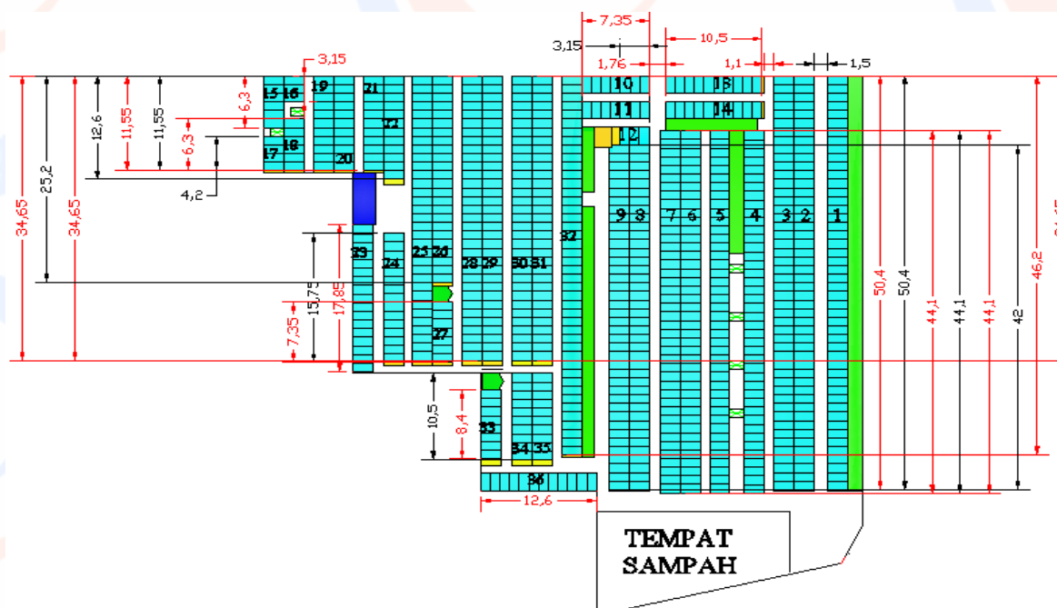
Gambar 5. Rancangan Model Area Parkir Belakang Modifikasi Kondisi Saat Ini (Sumber: Hasil Pengamatan dan Pengolahan, 2016)
