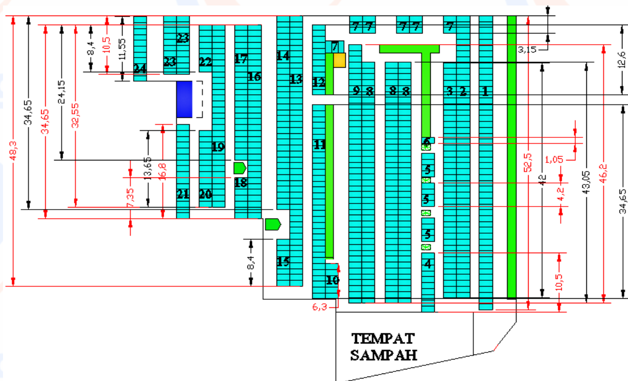
Gambar 6. Rancangan Model Area Parkir Belakang Pola Sudut 90° (Sumber: Hasil Pengamatan dan Pengolahan, 2016)
