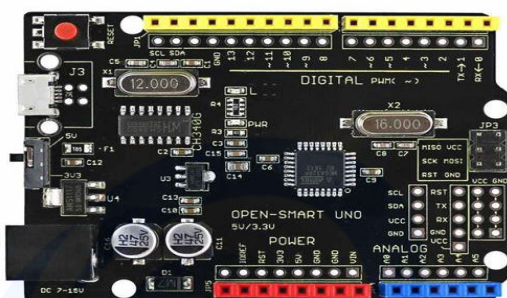
Gambar 2, Arduino Uno
