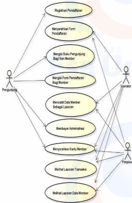
Gambar 3. Usecase diagram saat ini
