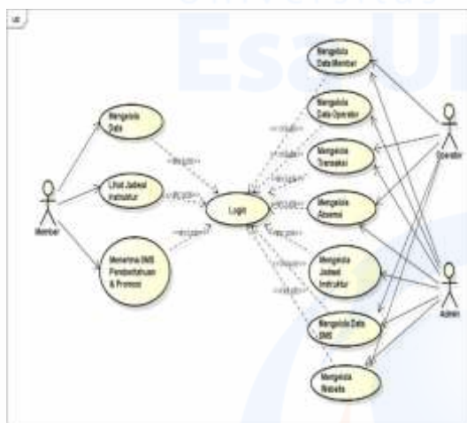
Gambar 4. Usecase diagram yang diusulkan
