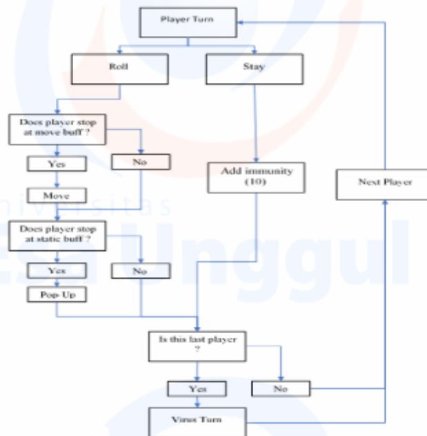
Gambar 3. Skema Alur Giliran Pemain
