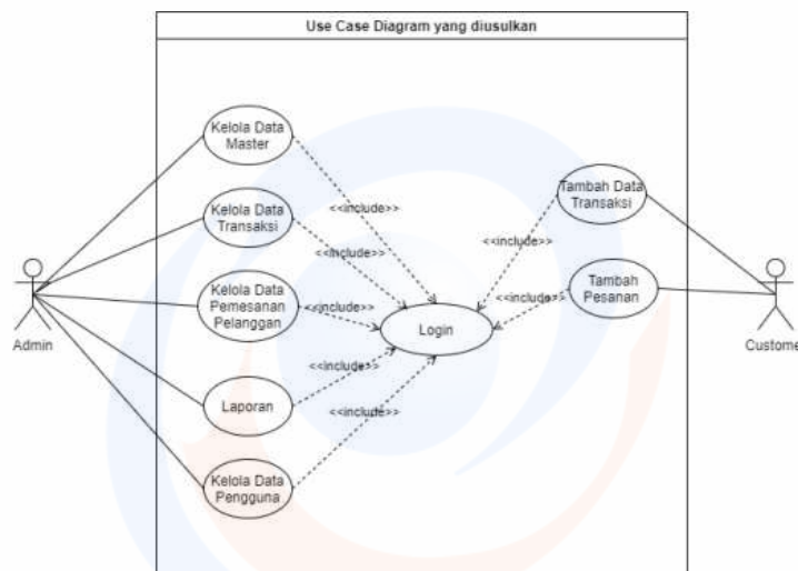
Gambar 4 Use Case Diagram yang diusulkan
