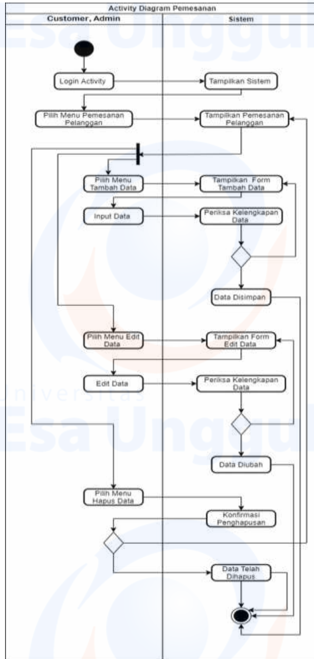
Gambar 5 Activiy Diagram Pemesanan
