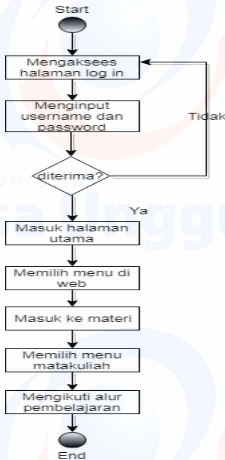
Gambar 1 Perancangan Aplikasi
