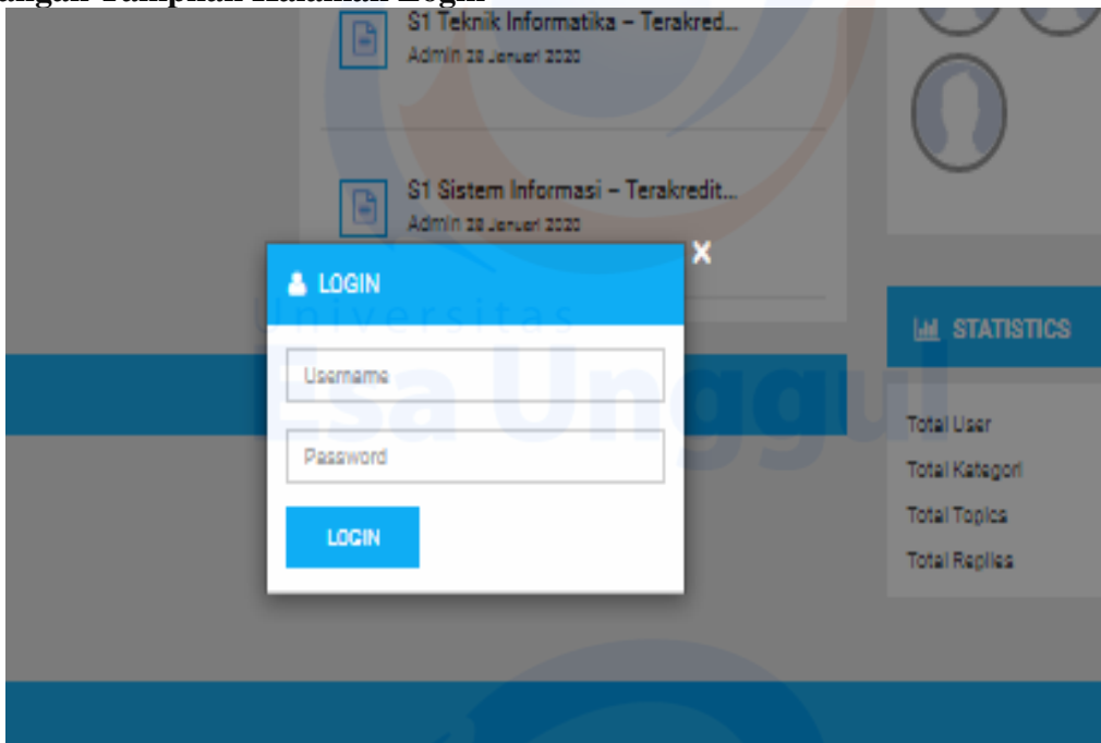
Gambar 3 Halaman Login
