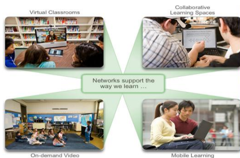
Gambar 1 Jaringan komputer
