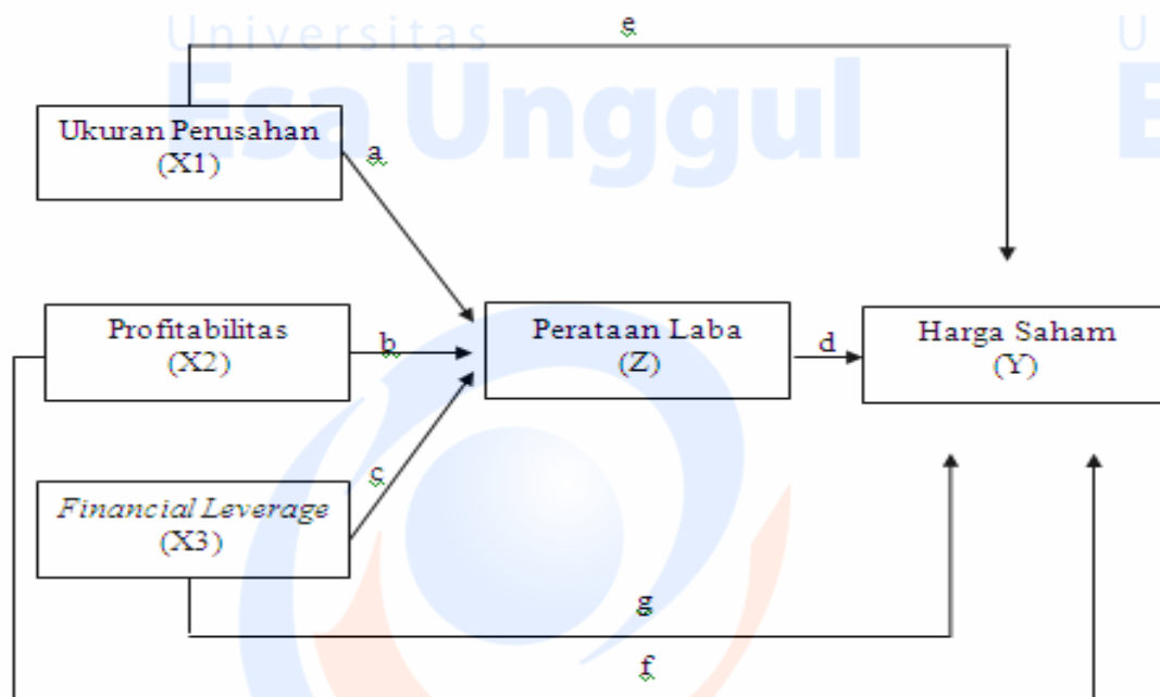
Gambar 4.2 Analisis Jalur
