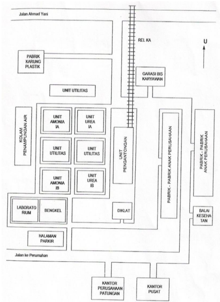
Lay out Pabrik PT Pupuk Kujang.
