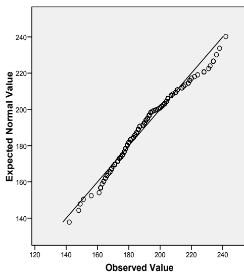
Normal Q-Q Plot of konsep_diri
