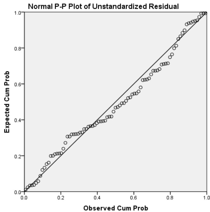
Gambar Hasil Uji Normalitas Grafik P-P Plot setelah Pembuangan Data Outlier
