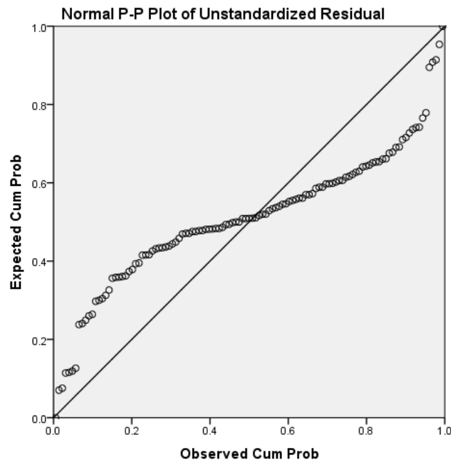
Gambar Hasil Uji Normalitas Grafik P-P Plot sebelum Pembuangan Data Outlier
