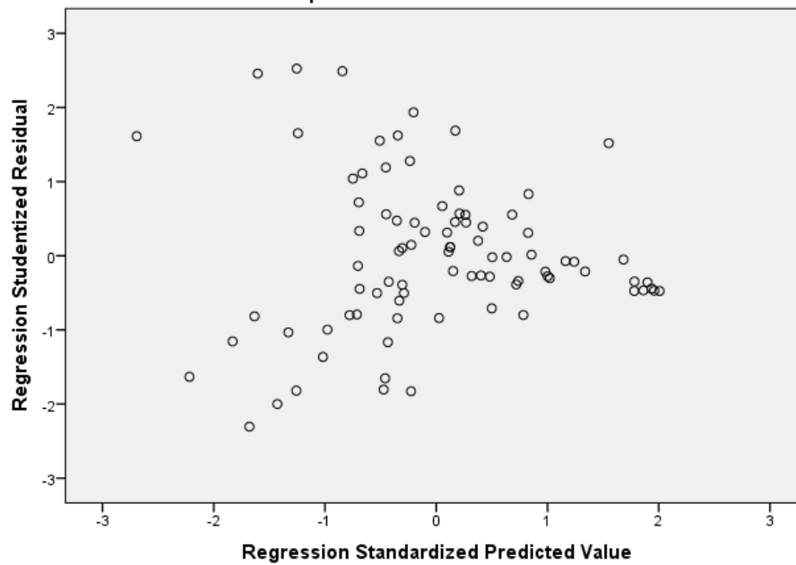
Gambar Hasil Uji Heterokedastisitas
