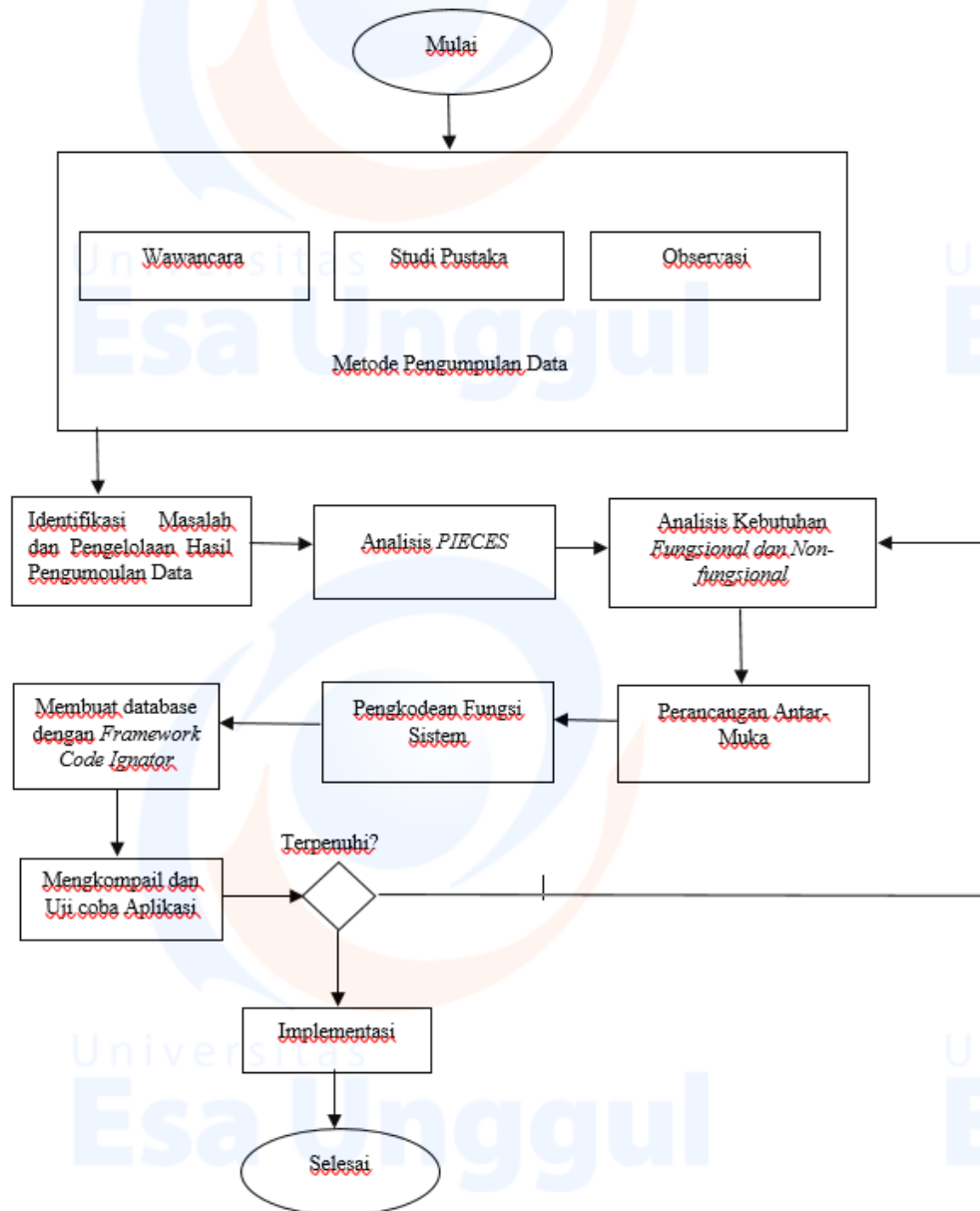
Gambar 1. Kerangka Berfikir
