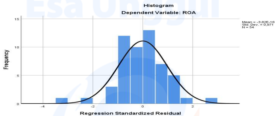
Gambar 3. Hasil Uji Histogram
