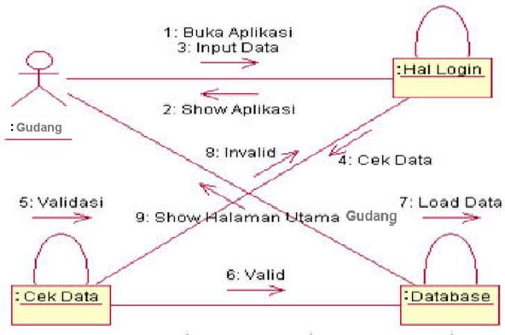
Collaboration Diagram Gudang Login. (Sumber : Penulis)
