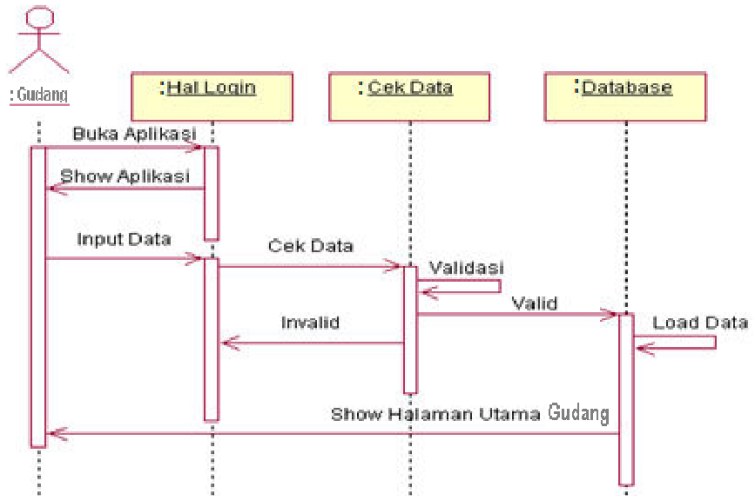
Sequence Diagram Login Gudang. (Sumber : Penulis)
