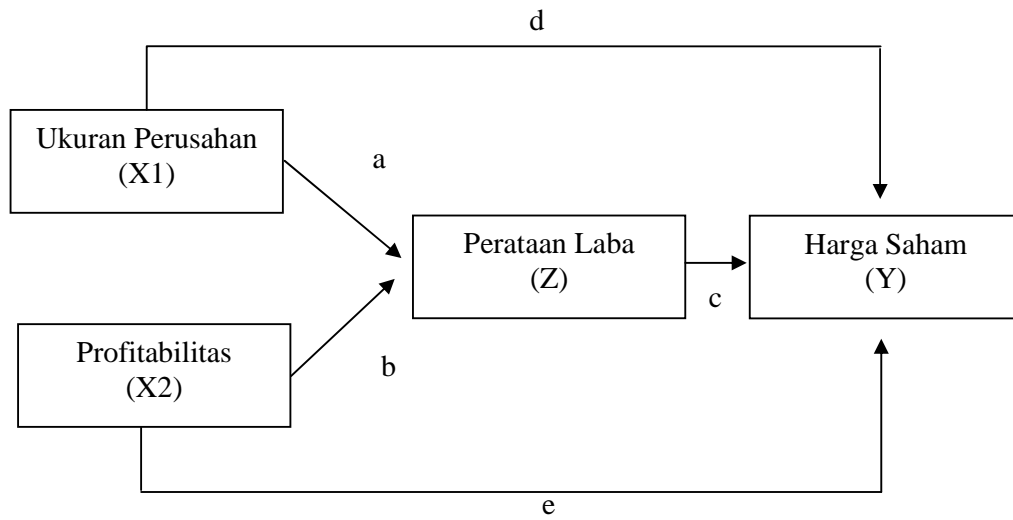
Gambar 4.2 Analisis Jalur
