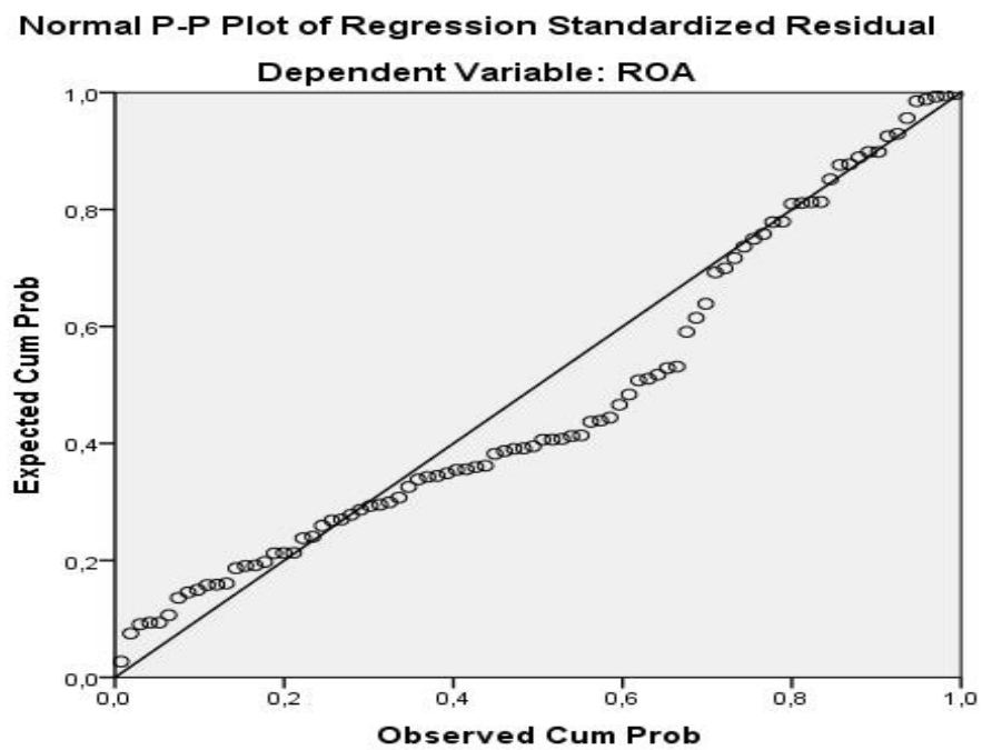
Gambar 4.1. Uji Normalitas Data ROA Sumber: Hasil Pengolahan Data SPSS 23, 2016
