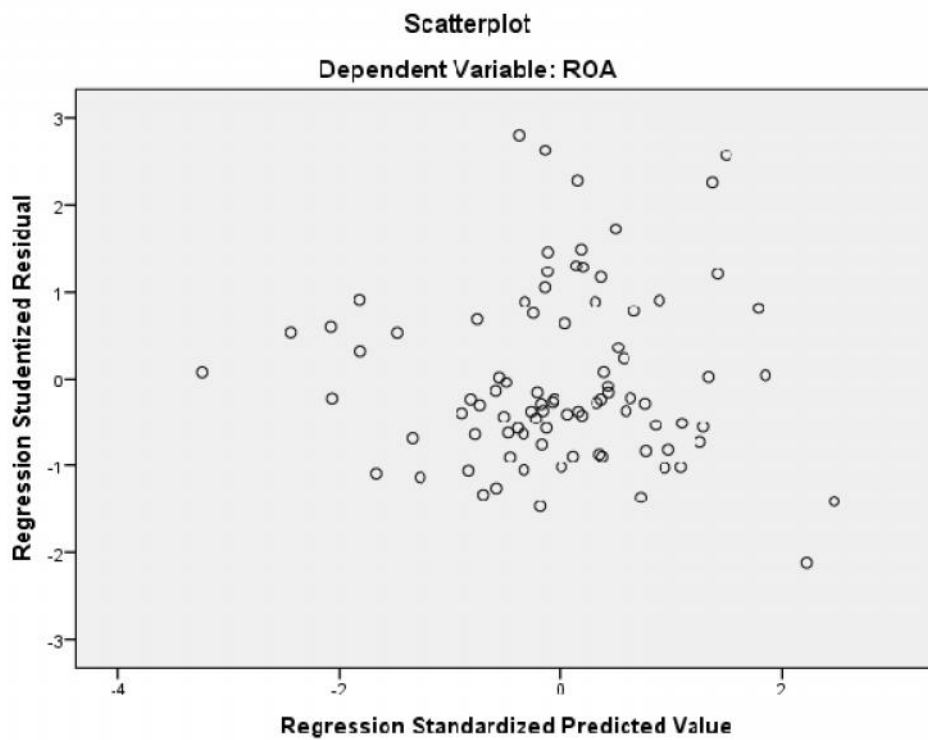
Gambar 4.3 Hasil Uji Heterokedasitas
