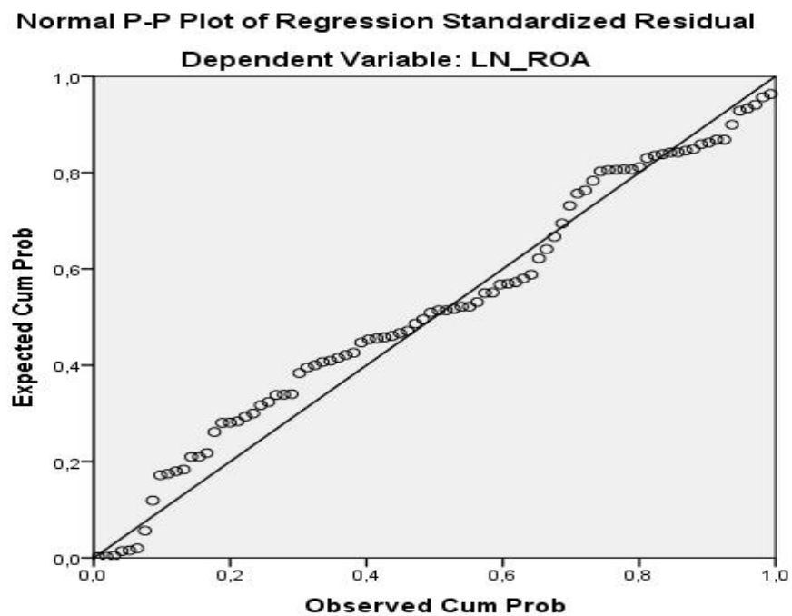
Gambar 4.2 Hasil Normalitas Data LN_ROA Sumber: Hasil Pengolahan Data SPSS 23, 2016
