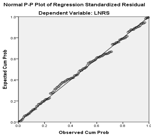
Gambar 4.1 Hasil Uji Normalitas Grafik Normal P-Plot (Ln)
