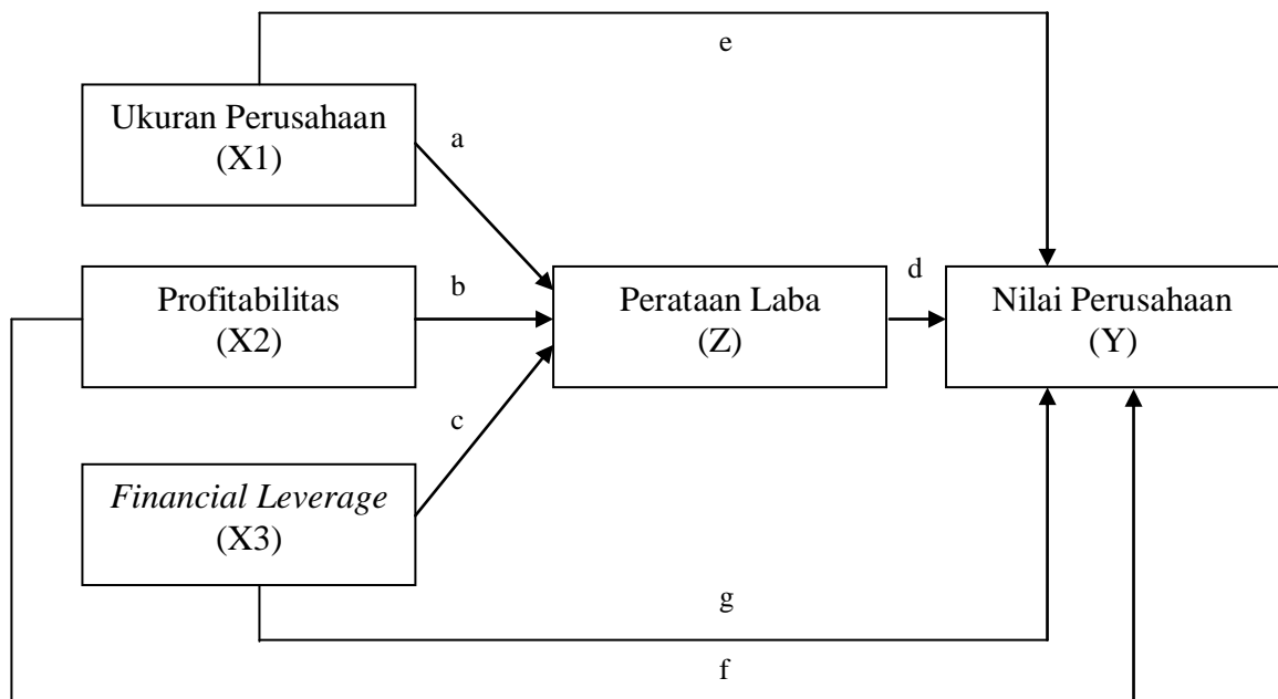
Gambar 4.2 Analisis Jalur
